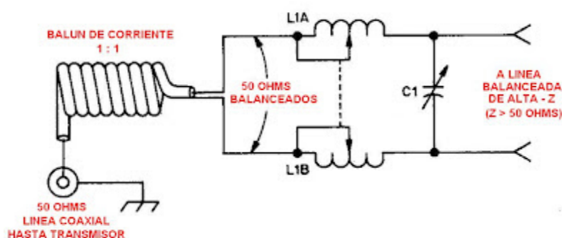
Ejemplo de acoplador en doble-L para línea balanceada.
